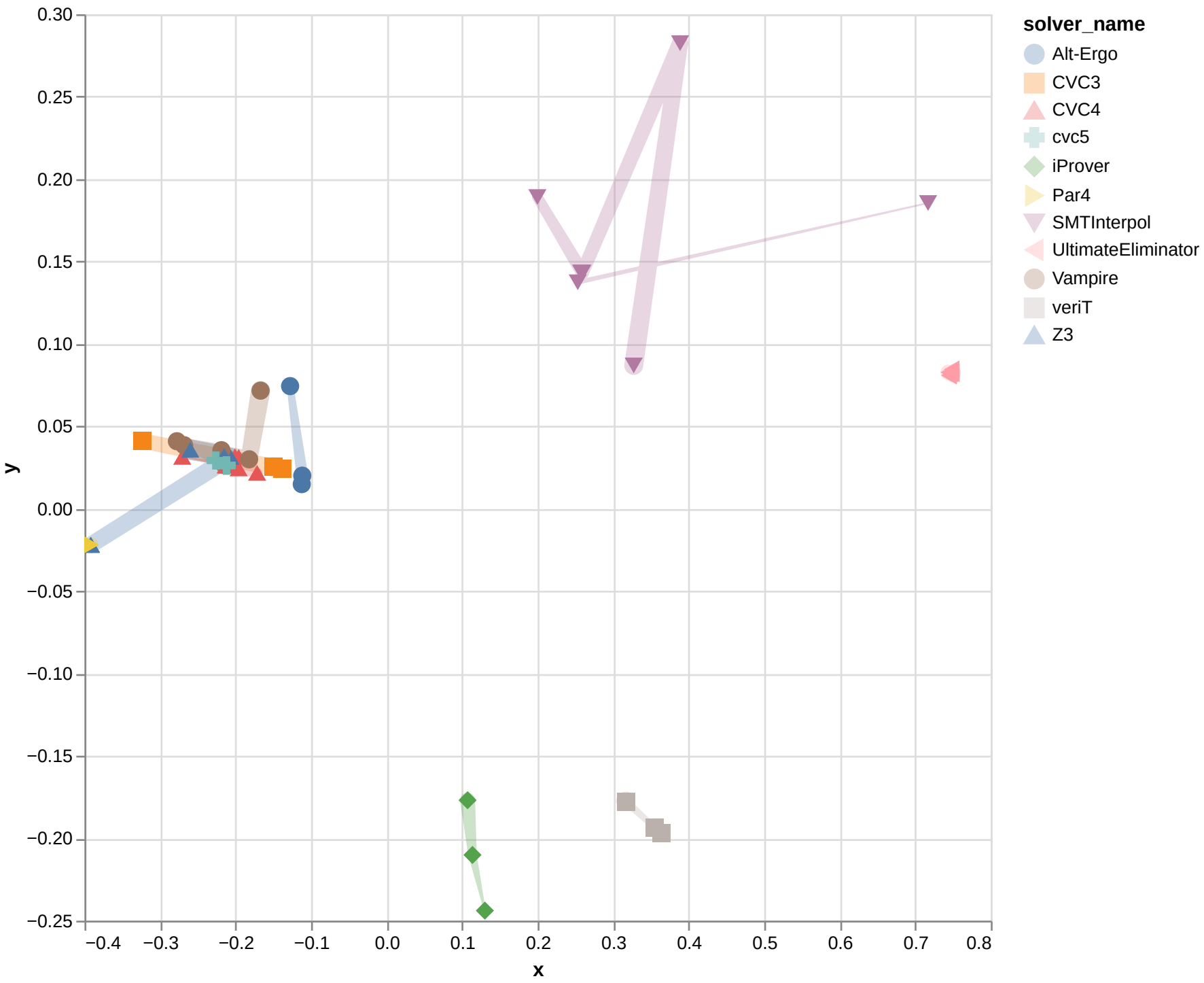
Isomap with cosine for AUFLIRA
