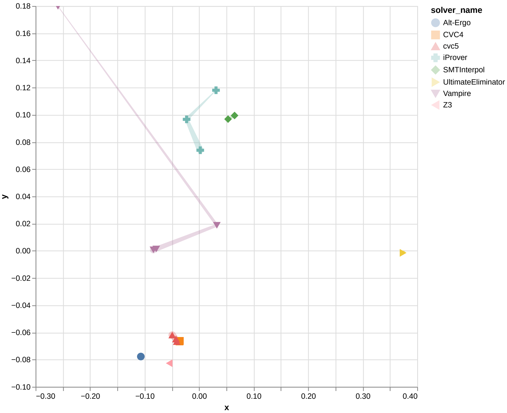
Isomap with cosine for AUFDTNIRA
