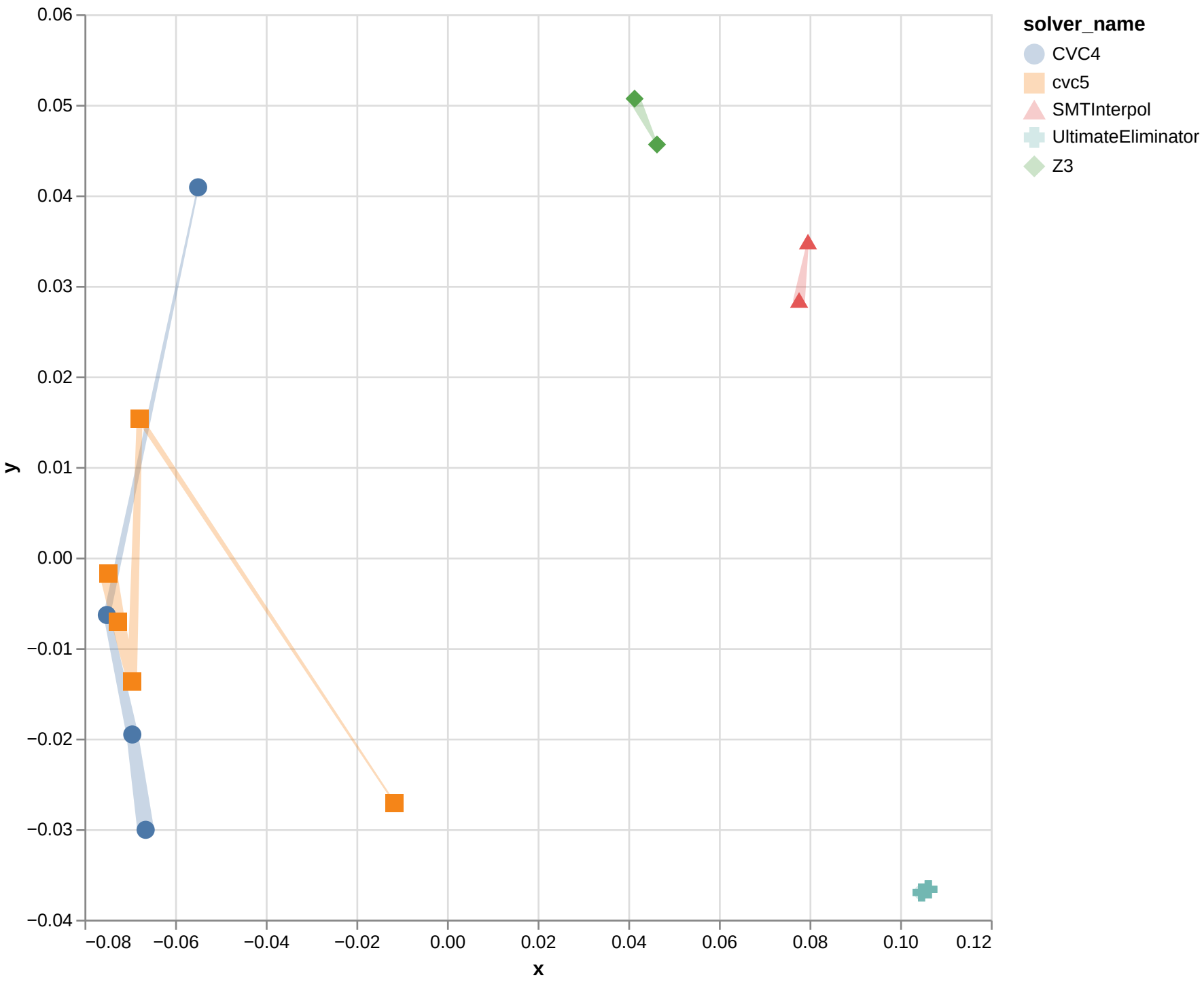
Isomap with cosine for AUFBVDTLIA
