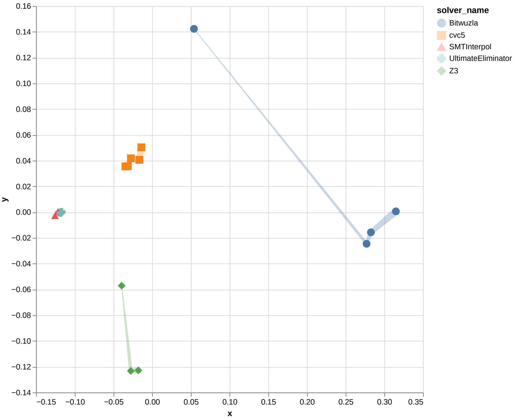
Isomap with cosine for AUFBV
